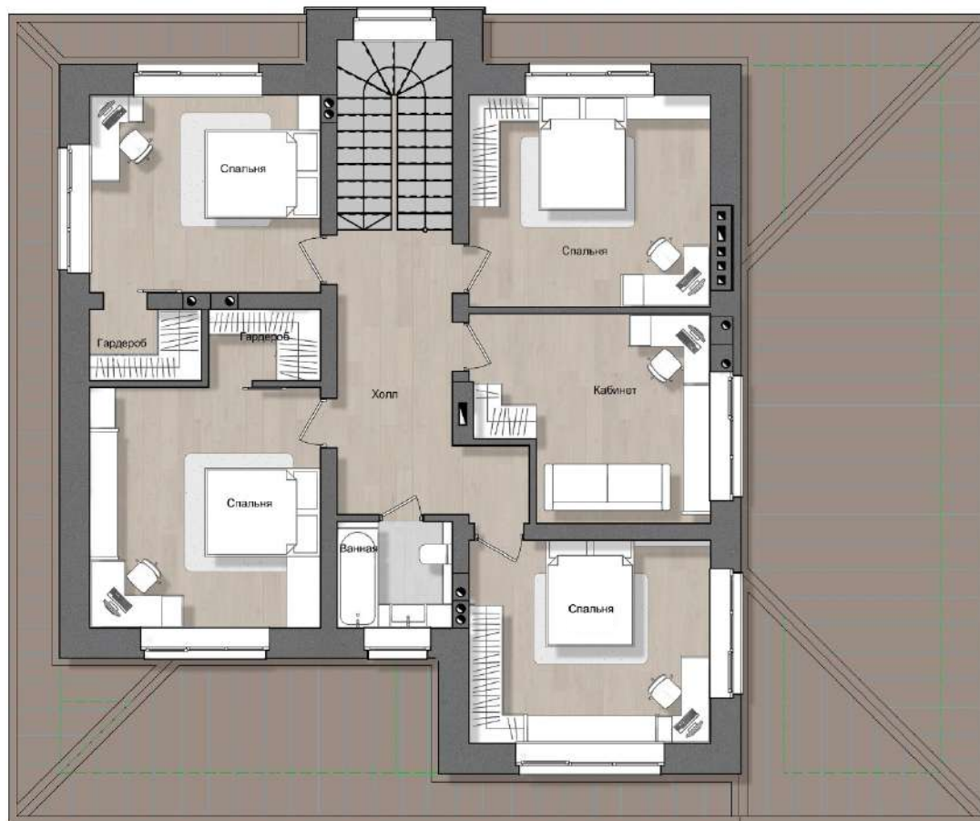
2 этаж
