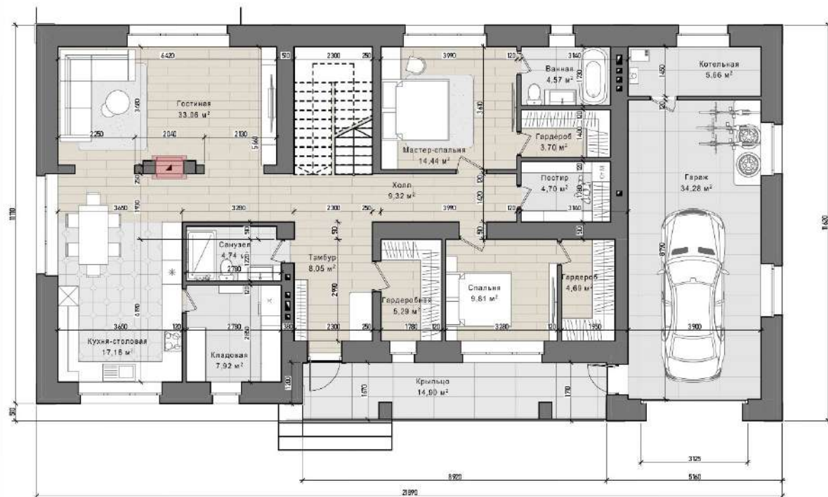
Планировка 1-го этажа
