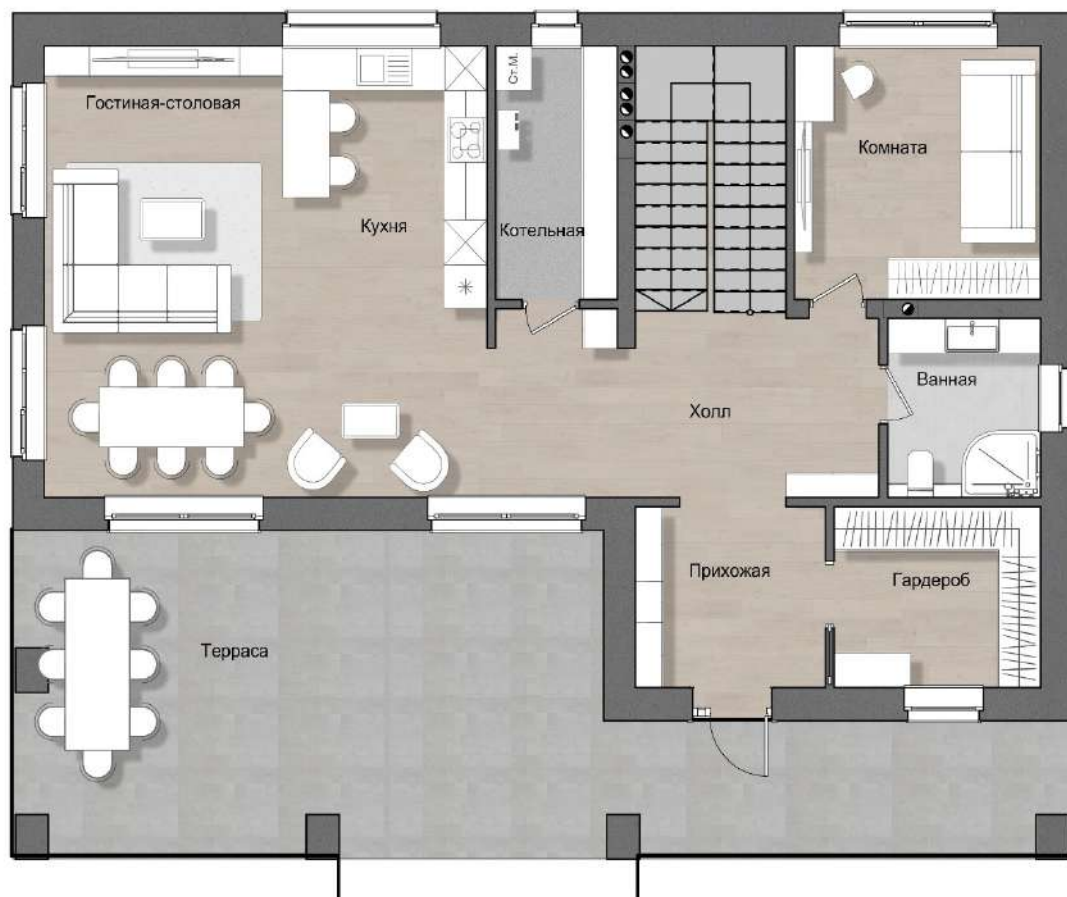
1 этаж
