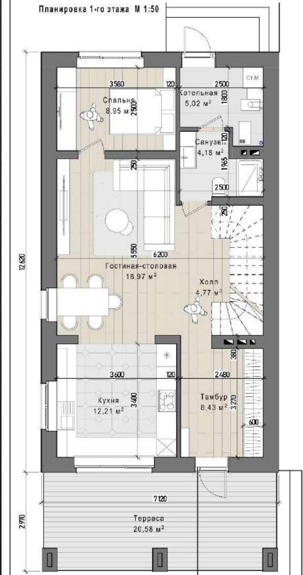
Экспликация помещений 1-го этажа
