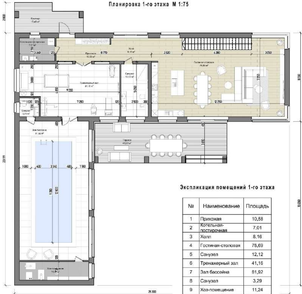
Планировка 1-го этажа М 1:75
